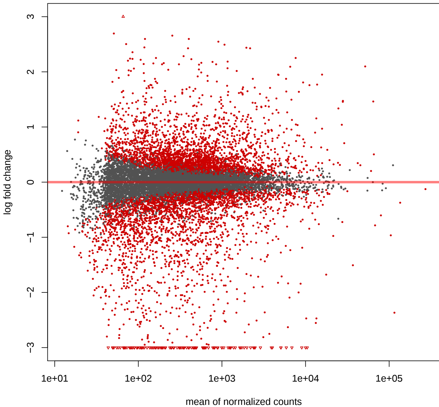
DESeq2 MA plot
